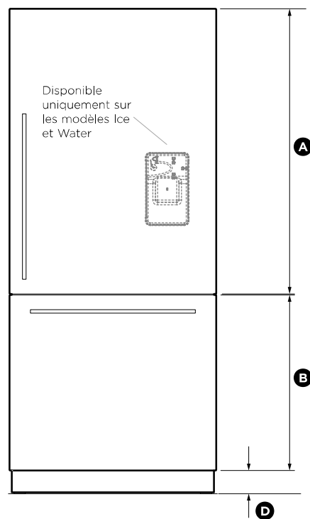
ENSEMBLE DE PANNEAU DE PORTE RD3680
