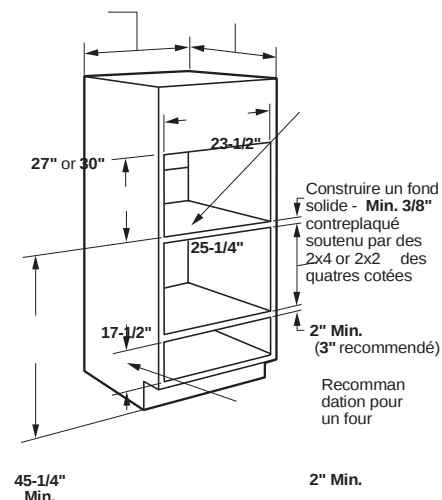
Installation sur un four mural et un tiroir réchaud:
