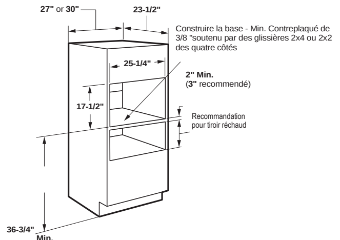
Installation sur un four mural et un tiroir réchaud:
