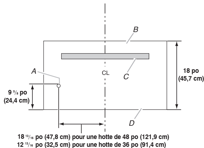
VUE ARRIÈRE
