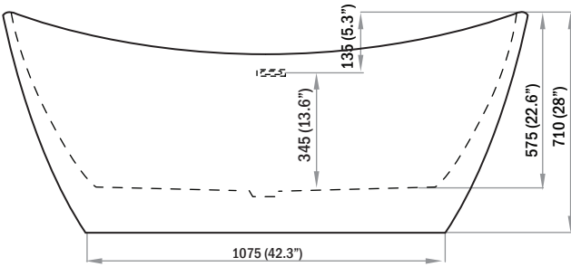
FRONT VIEW VUE DE FACE
