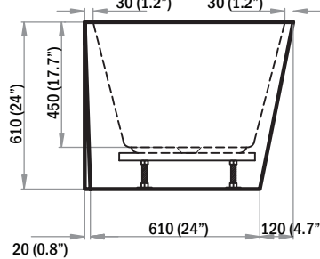
SIDE VIEW VUE DE CÔTÉ
