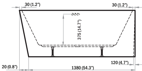
FRONT VIEW VUE DE FACE
