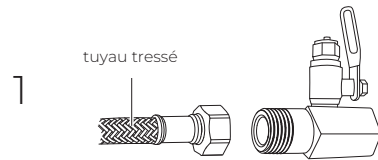
Tuyau tressé en acier inoxydable 1/2 BSP avec filetage 7/16-24 UNS (1x)
