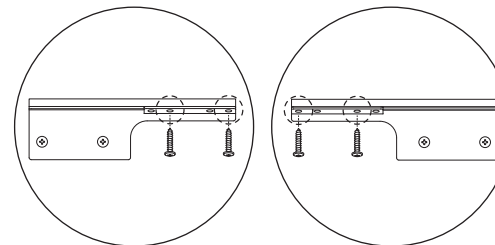
Support supérieur gauche
