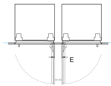
CHARNIÈRE À CHARNIÈRE Permettant d'ouvrir les deux portes en même temps - nécessite un espace entre les modèles
