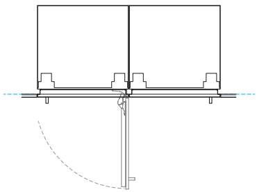
CHARNIÈRE À CHARNIÈRE Permettant d'ouvrir une seule porte à la fois
