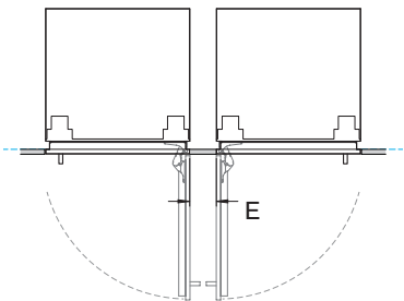
CHARNIÈRE À CHARNIÈRE Permettant d'ouvrir les deux portes en même temps - nécessite un espace entre les modèles
