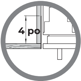
FINITION SUR LES CÔTÉS ET DANS LE HAUT DE LA CAVITÉ
