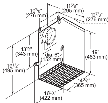
DHR1FZUC Ventilateur externe 600 PCM
