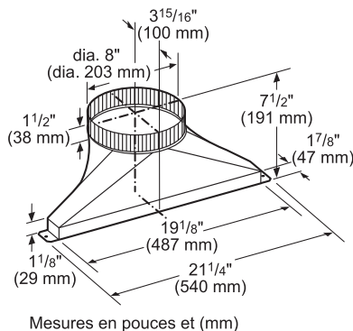
Mesures en pouces et (mm)
