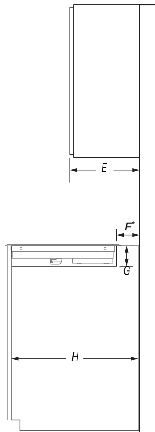
VUE LATÉRALE
