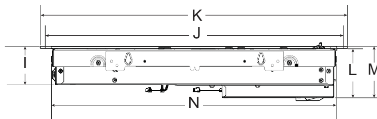
VUE LATÉRALE
