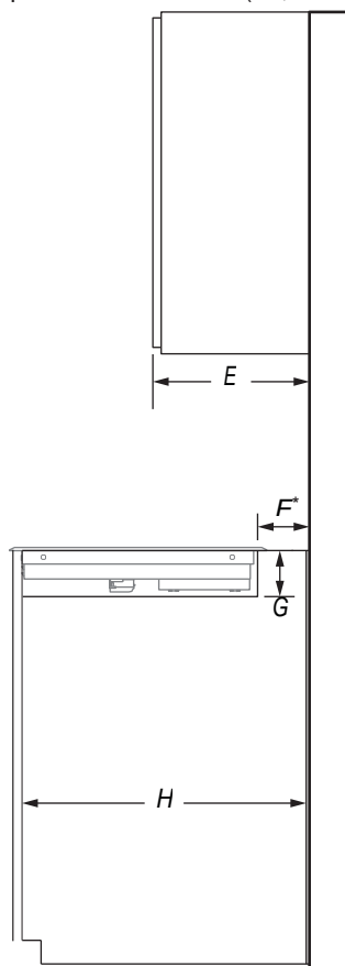
VISTA LATERAL
