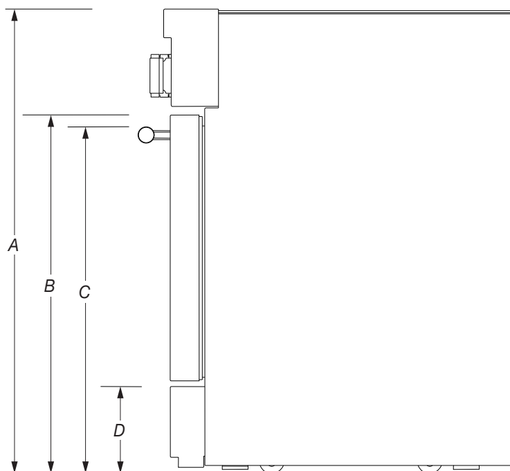
VUE LATÉRALE
