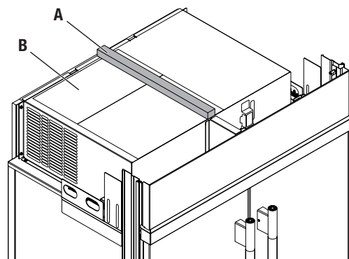
A. Gasket
